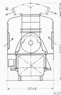
Bild 7. Fahrbare Gasturbinen-Zentrale von 3000 kW
