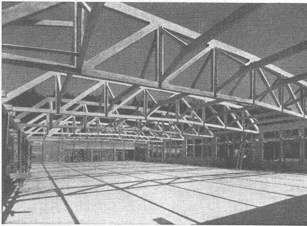
Eisenbetonfachwerk - Montagefertig
