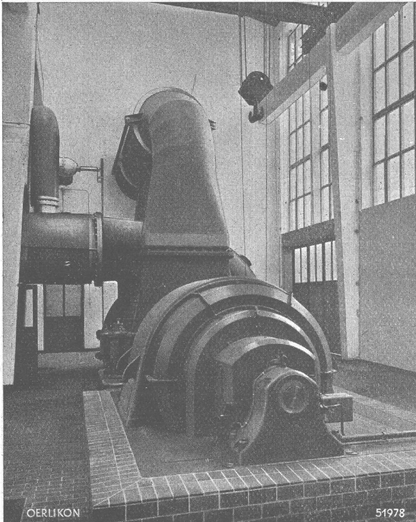
Die grösste Wärmepumpe der Welt - mit elektrischem Antrieb OERLIKON
