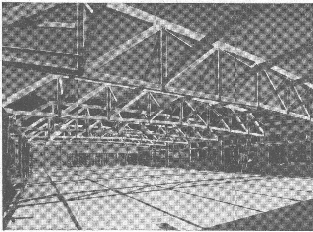
Eisenbetonfachwerk - Montagefertig
