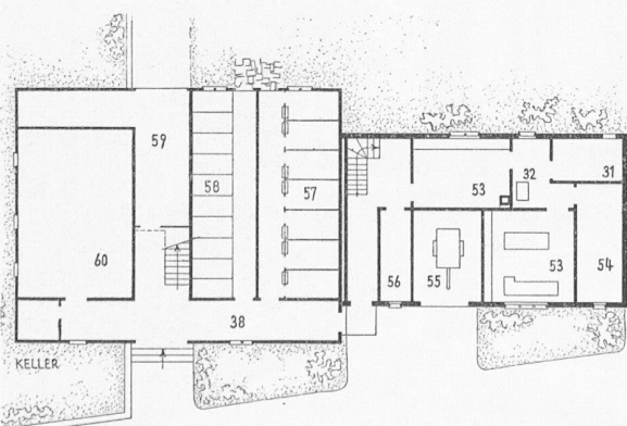
Bilder 47 bis 49. Altes Bauernhaus (16), Grundrisse 1:400
