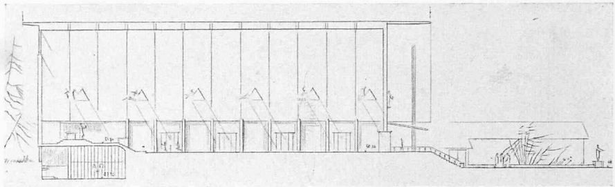
Längsschnitt 1: 600
