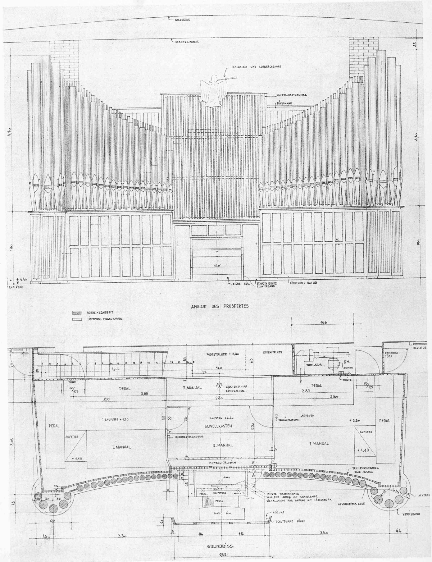
Bild 5. Werkzeichnung der Orgel, verkleinert auf den Masstab 1 : 60. Die Orgel, gebaut von der Firma Th. Kuhn A.-G. in Männedorf, hat 29 klingende Stimmen und zwei Pedaltransmissionsregister, zwei Manuale und ein Pedal. Experte für Orgel und Geläute war Prof. Ernst Schiess, Bern
