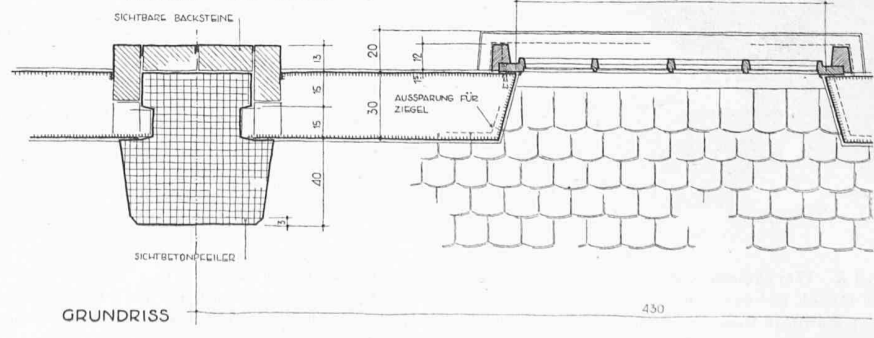
Bild 4. Einzelheiten der Konstruktion und der architektonischen Gestaltung. Masstab 1: 33
