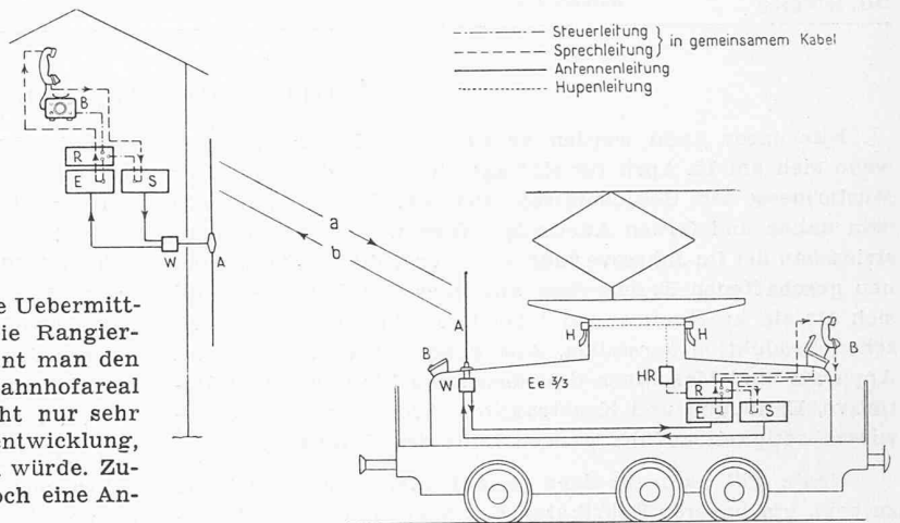
Bild 3. Aufbau der Rangierfunkanlage
