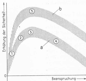
Bild 2. Erhöhung der Sicherheit der Zugführung und Beanspruchung des Führers durch Sicherheitssteuerungen. a. Bereich bestehender Sicherheitssteuerungen mit Pedal, b. Bereich der neuen Sicherheitssteuerung, 1 bis 5 Pedalanordnungen gemäss Bild 1
