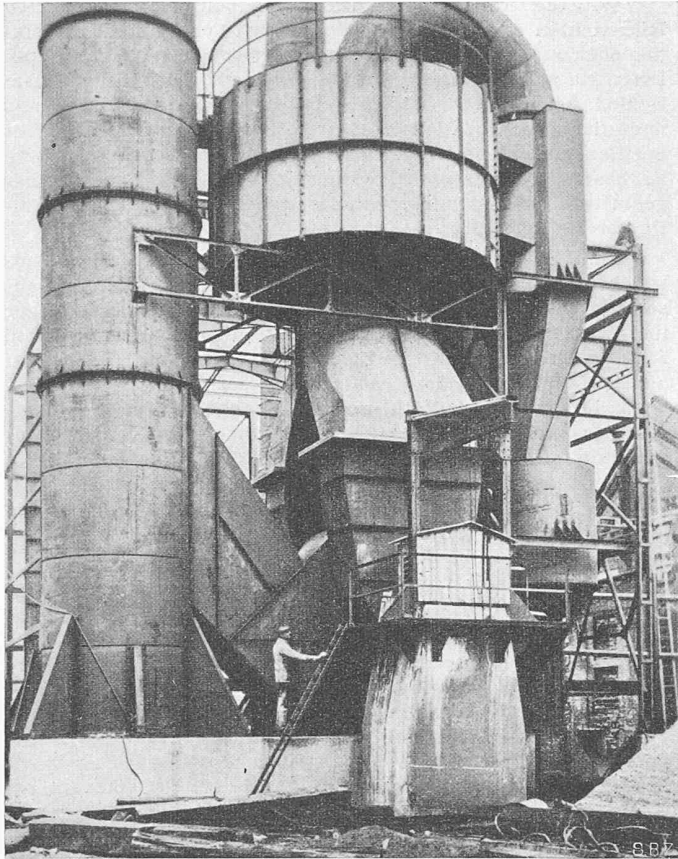
Bild 7. Doppelabscheider von Tonçeren, 252 kg/h Staub, Gasdurchsatz 232 000 m 3 /h, Gesamtstaubungsgrad 87 %
