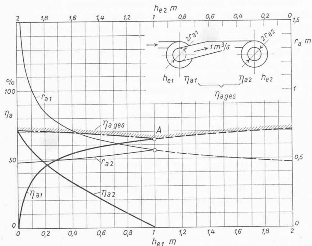
Bild 3. Der Anteil zweier in Reihe geschalteter Zyklone am Gesamtdruckverbrauch bestimmt die Zyklongrösse und den Wirkungsgrad
