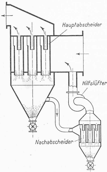
Bild 8. Im Duplex-Collector (Prat Daniel Corp.) regelt ein Hilfslüfter den Unterdruck im Staubsammelraum des Hauptabscheiders: ein Nachabscheider hält die Staubrückgabe aus dem Teilstrom in den Rohgaseintritt des Hauptabscheiders in zulässigen Grenzen
