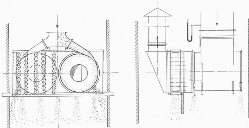
Bild 4. Zyklone in Reihenschaltung, mit Ueberdruck arbeitend (Wagner-Birò A.-G., Wien und Graz); unten Bild 5 Ansicht
