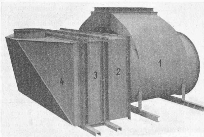
Bild 4. Zyklone in Reihenschaltung, mit Ueberdruck arbeitend (Wagner-Birò A.-G., Wien und Graz); unten Bild 5 Ansicht
