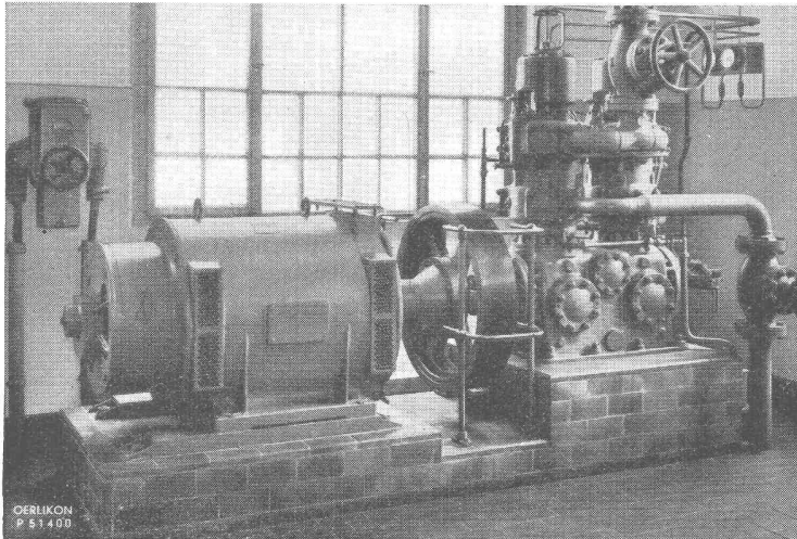
Kompressor, angetrieben durch Combi-Motor 95 kW, 380 V, 50 Hz.
