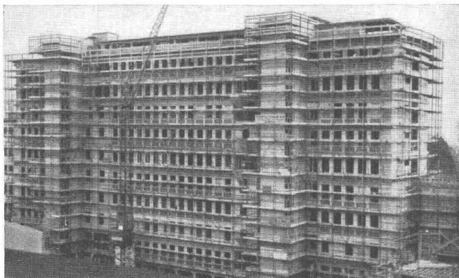
Bau- und Putzgerüst auf Konsolen, 35 m hoch
