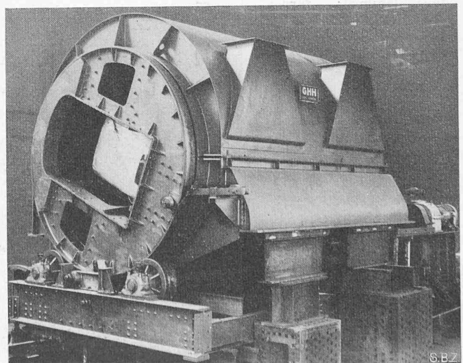
Bild 28. Kreiselschwinger
