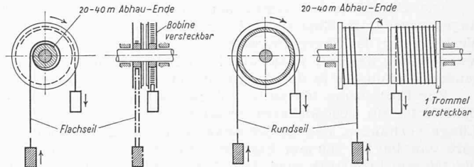
Bild 32a. Bobine Seilträger an Hauptschacht-Fördermaschinen Bild 32b. Zylindertrommel
