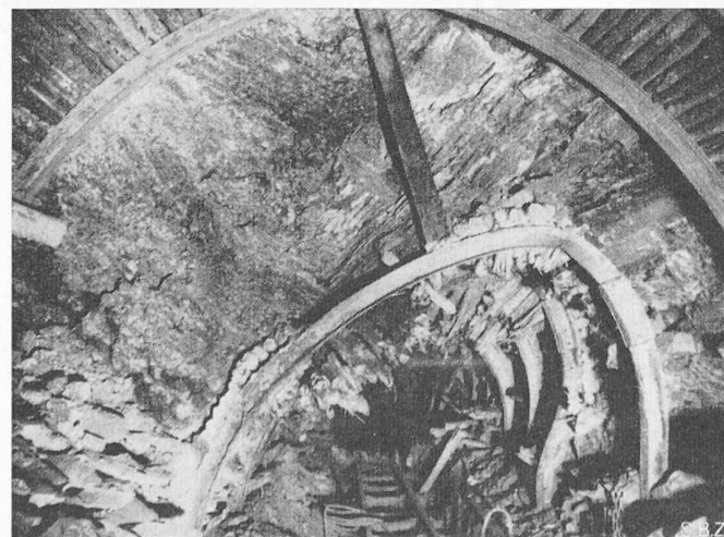
Bild 19. Aussermittige Auffaltung
