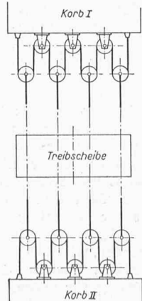
Bild 34. Ketten-Ausgleichvorrichtung
