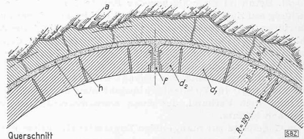
Bild 3. Einzelheiten der Auskleidung mit gemauertem Kernring
