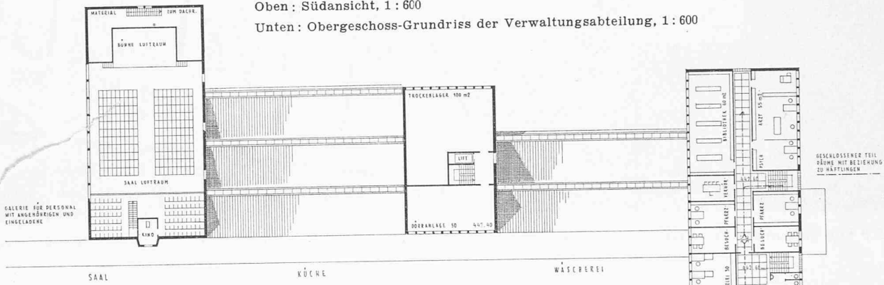
Oben: Südsicht, 1 : 600
