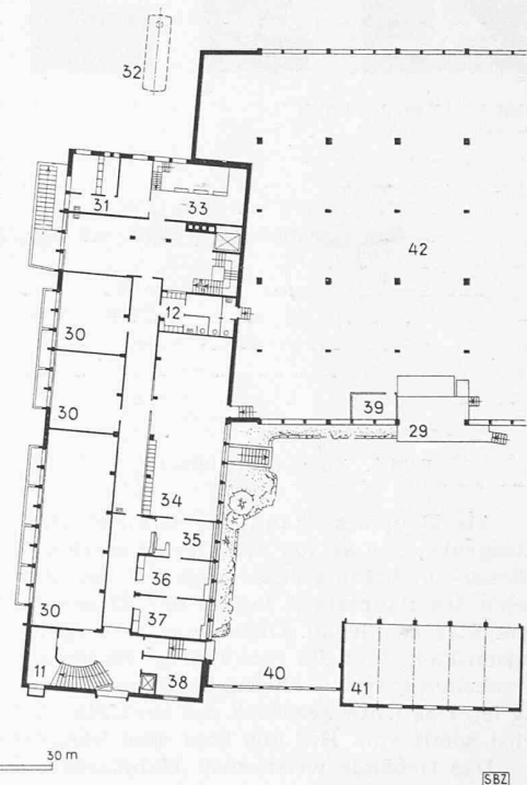
Bild 3. Untergeschoss, 1:700
