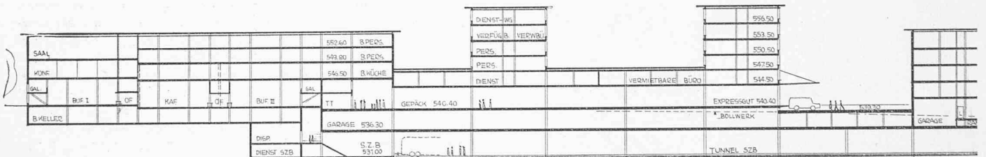
Längsschnitt entlang des Bollwerks, Masstab 1 : 1000
