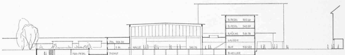
Querschnitt durch die Bahnhofhalle 1 : 1000
