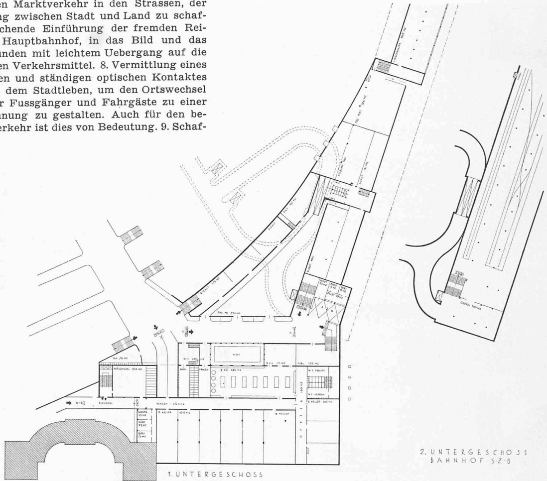
1. Untergeschoss des Aufnahmegebäudes, daneben 2. Untergeschoss, Masstab 1 : 1500
