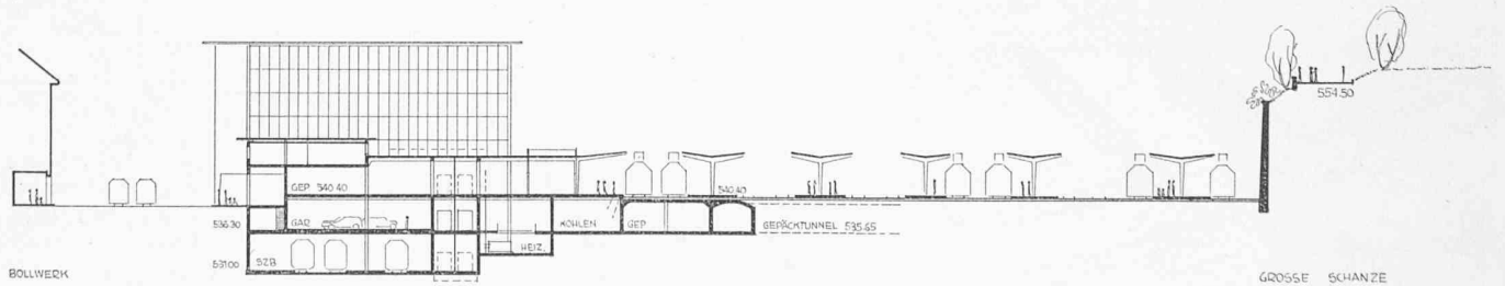
Schnitt quer zum Bollwerk durch die Gepäckexpedition, Gleisanlage und grosse Schanze, Masstab 1 : 1000
