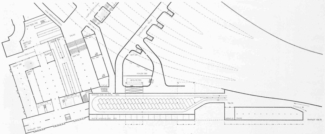
1. Untergeschoss, Masstab 1 : 1500
