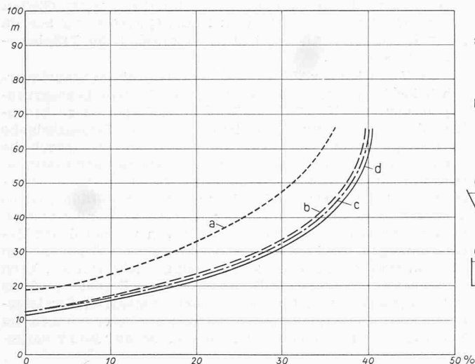
Bild 3. Erzielbare Einsparung an Betonvolumen bei Anwendung einer Staumauer in aufgelöster Bauweise, Typ «Bau Muggers», im Vergleich zu einer gleich hohen, massiven Gewichtsstaumauer bei verschiedenen Talprofilen (a, b, c, d). Ordnate: Mauerhöhe bis Stauspiegel in m; Abszisse: Prozentuale Einsparung für die aufgelöste Staumauer
