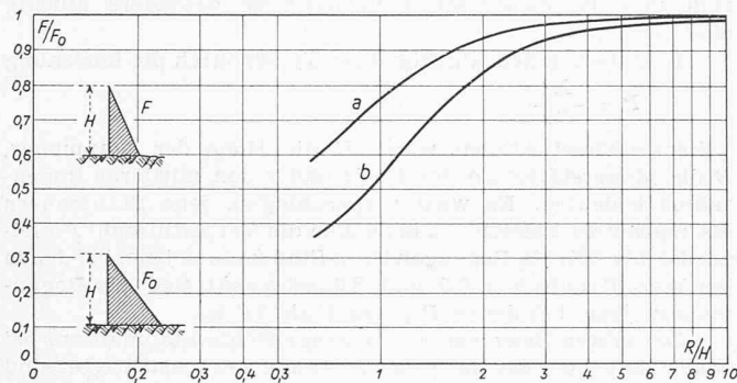
Bild 4. Vergleich zwischen Bogengewichts-Staumauer und massiver Gewichtsstaumauer. Ordnate: Verhältnis der Querschnittsflächen F/F_0 ; Abszisse: Verhältnis R/H nach Tölke ( R Krümmungsradius im Schwerpunkt des Mauerquerschnitts, H Höhe der Staumauer). F Querschnitt einer Bogengewichts-Staumauer, F_0 Querschnitt einer massiven Gewichtsstaumauer. a Verhältnis F/F_0 bei starrem Untergrund ( E = \infty ). b Verhältnis F/F_0 bei elastischem Untergrund (gleicher Elastizitätsmodul wie bei Beton nach Young)
