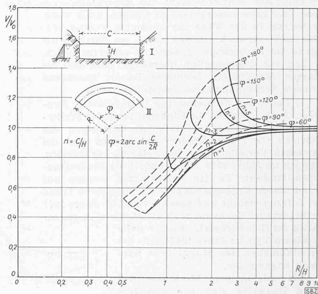
Bild 6. Vergleich zwischen Bogengewichts-Staumauer und massiver Gewichtsstaumauer bei U-Profil.
