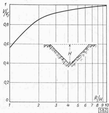
Bild 5. Vergleich zwischen Bogengewichts-Staumauer und massiver Gewichtsstaumauer bei V-Profil. Ordnate: Verhältnis der Volumina V/V_0 ; Abszisse: Verhältnis R/H
