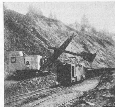
Bild 5. Laden in einem Tagbau mit Bagger von 1 m 3 Löffelinhalt
