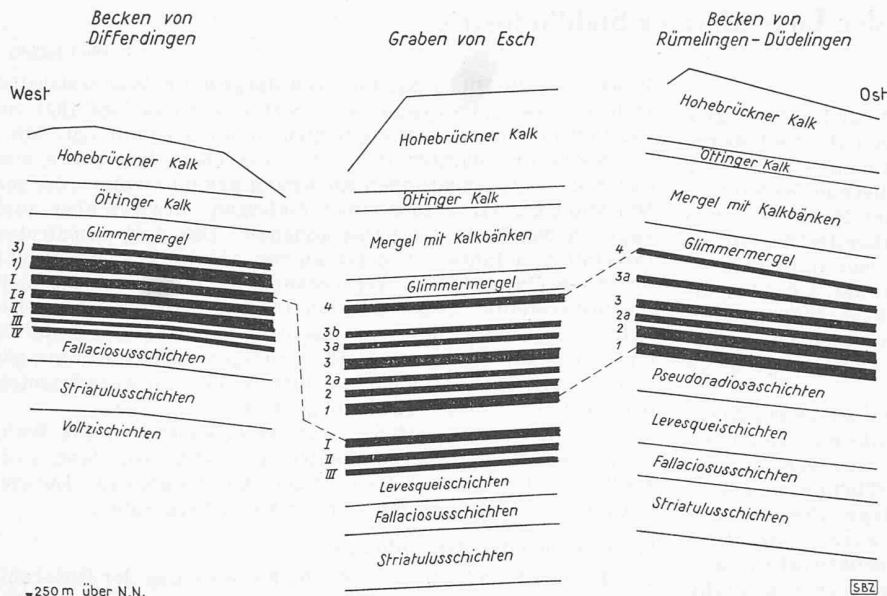
Bild 4. Stratigraphische Gegenüberstellung der verschiedenen Becken Masstab der Höhen rd. 1:3000. Legende der Schichtbezeichnungen siehe Bild 2
