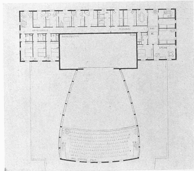
Obergeschoss 1:600
