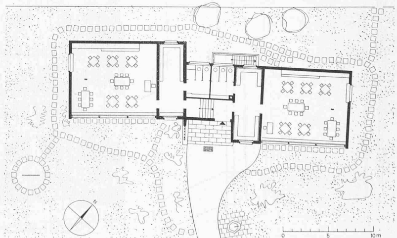
Bild 3. Grundriss 1:400
