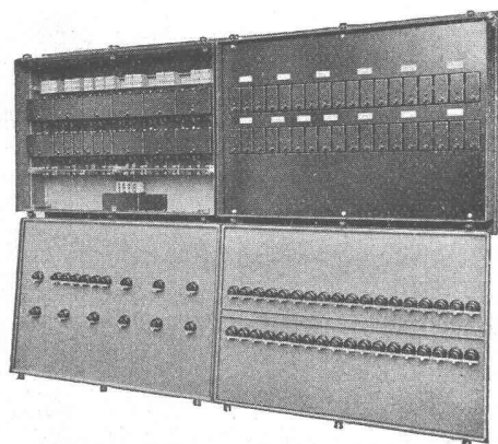
Verteilkasten mit CMC-Kleinautomaten (Kastentüren herabgeklappt)
