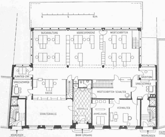
Bild 11. Erdgeschoss 1:350 gemäss Ausführung
