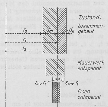
Bild 3. Erklärungsskizze zur Vorspannung
