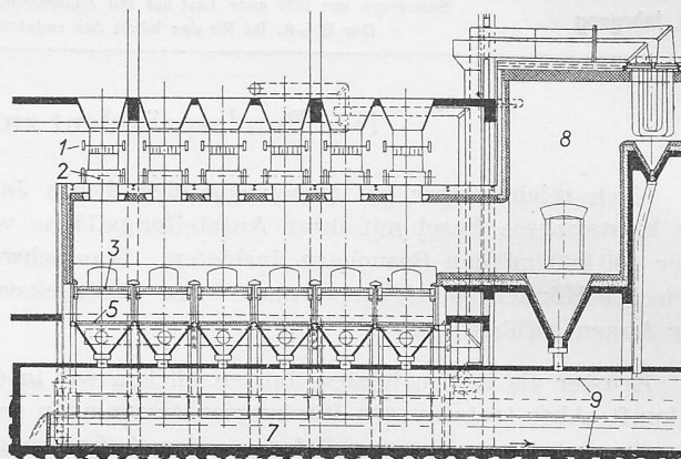
Bild 1. Längsschnitt durch einen Zellenofen, Masstab 1:300. 1 Dosiervorrichtung, 2 verschiebbarer Einfülldeckel, 3 Planrost, 4 Tür, 5 Schlackenrost, 6 Räumler, 7 Schlackenkanal, 8 Verbrennungskammer, 9 Kratzerkette
