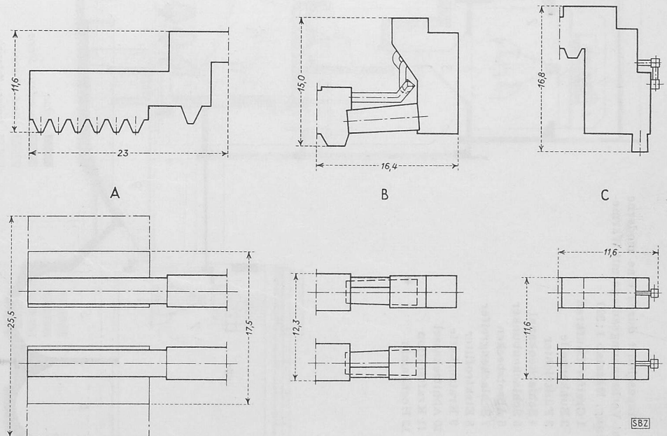
Bild 5. Vergleich der Ofenabmessungen verschiedener Systeme, Durchsatzmenge 2 \times 200 t/24 h A Zellenofen, B kontinuierlicher Ofen, C von Roll-Ofen
