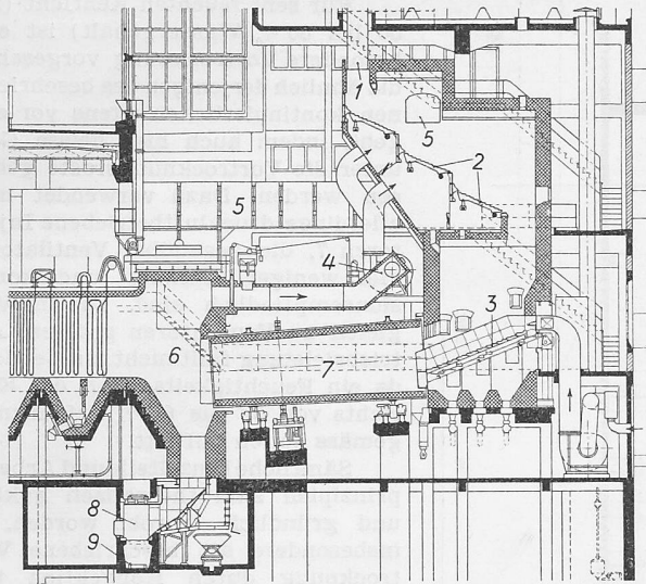
Bild 3. Längsschnitt durch einen kontinuierlich arbeitenden Ofen mit Gas-Rücksaugung, Masstab 1 : 300 (Beschreibung s. [2]) 1 Einfüllschacht, 2 Vortrocknungsroste, 3 Anzündrost, 4 Rauchgas-Ventilatoren, 5 By-pass Kanal, verbindet Raum 6 mit Raum über 2, 6 Verbrennungskammer, 7 Drehtrommel, 8 Schlackenkanal, 9 Kratzerkette
