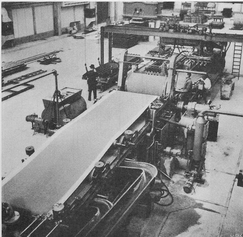
Bild 3. Plattenmaschine von oben; am hintern Ende des Filzbandes die Formatwalze, dahinter die Abhebevorrichtung, im Hintergrund die Presse
