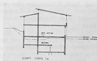
Schnitt Ia, 1:600
