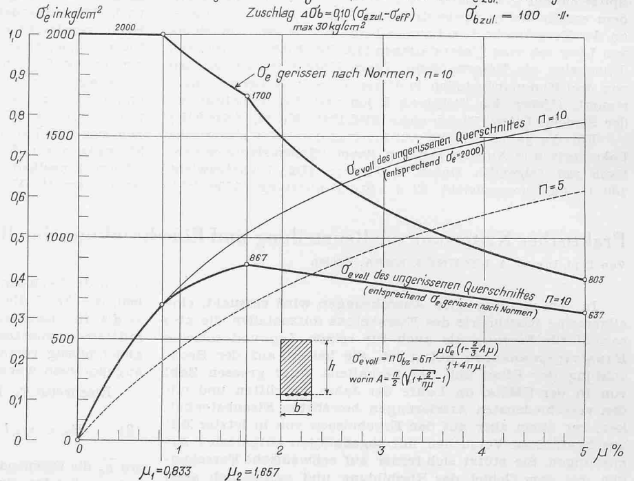
Bild 2. Rechteckquerschnitt. Rechnerische Zugspannungen der Stahleinlagen im vollen und im gerissenen Querschnitt unter der Nutzlast
