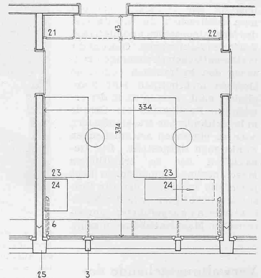
Bild 6. Bureau-Grundriss 1:70
