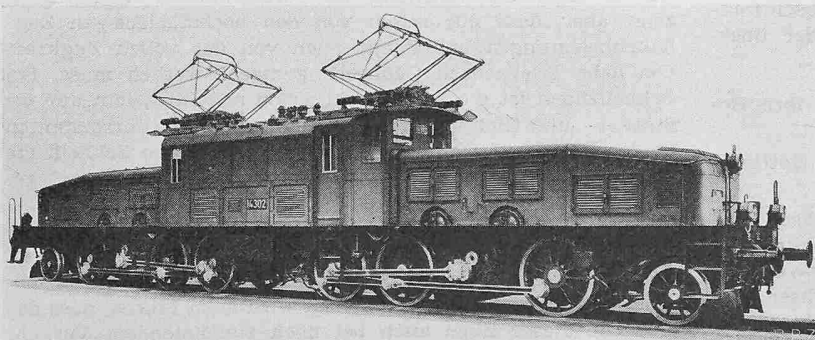
Bild 1. Lokomotive Ce 6/8: Baujahr 1925-27 (frühere Serie 1919-22), Stundenleistung 2460 PS bei 35 km/h, Höchstgeschwindigkeit 65 km/h, Gewicht 131 t, Reibungsgewicht 109 t
