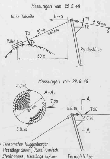
Bild 12b. Anordnung der Messinstrumente am Tragseil des Kabelkrans K_3
