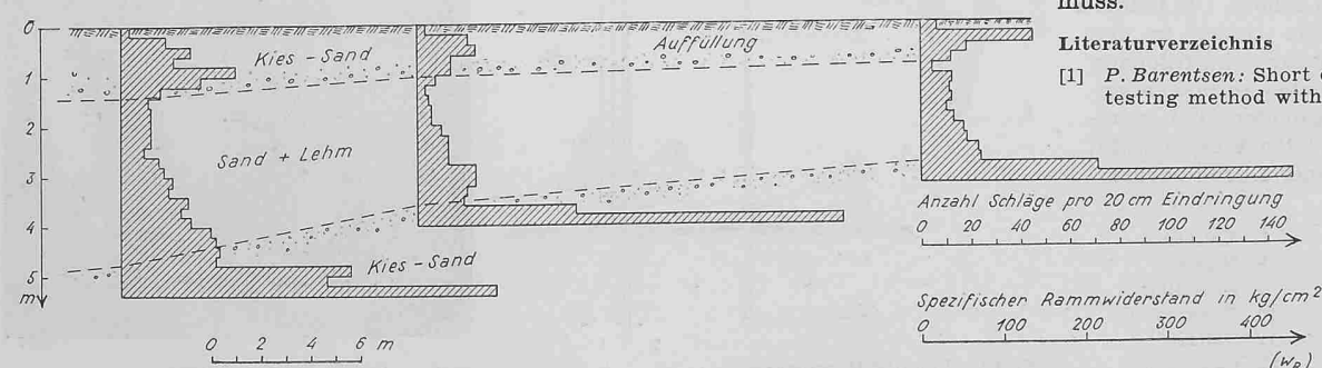
Bild 13. Ermittlung des Aufbaues eines alten Flussdamms
