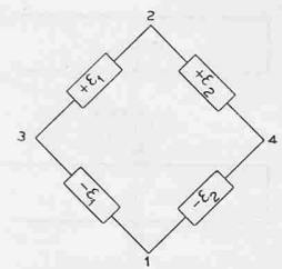
Bild 4. Messbrücken-Schaltung für die Bestimmung von Schubkräften
