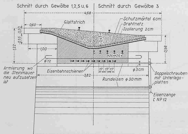
Bilder 5 und 6. Schmalztobel-Viadukt. Querschnitte durch den Brückentrog, 1:80
