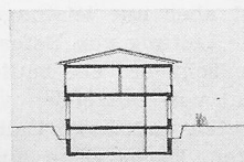
Schnitt Mittelbau
