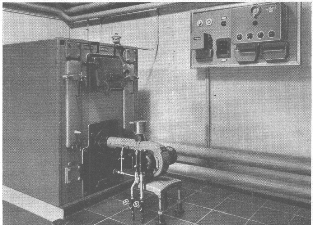
Im Mehrfamilienhaus automatische Gruppensteuerung, ausgestattet mit Aussentemperaturregler-Anlage
