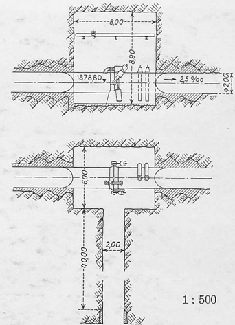
Bild 15. Apparatekammer im Mauerblock 24
