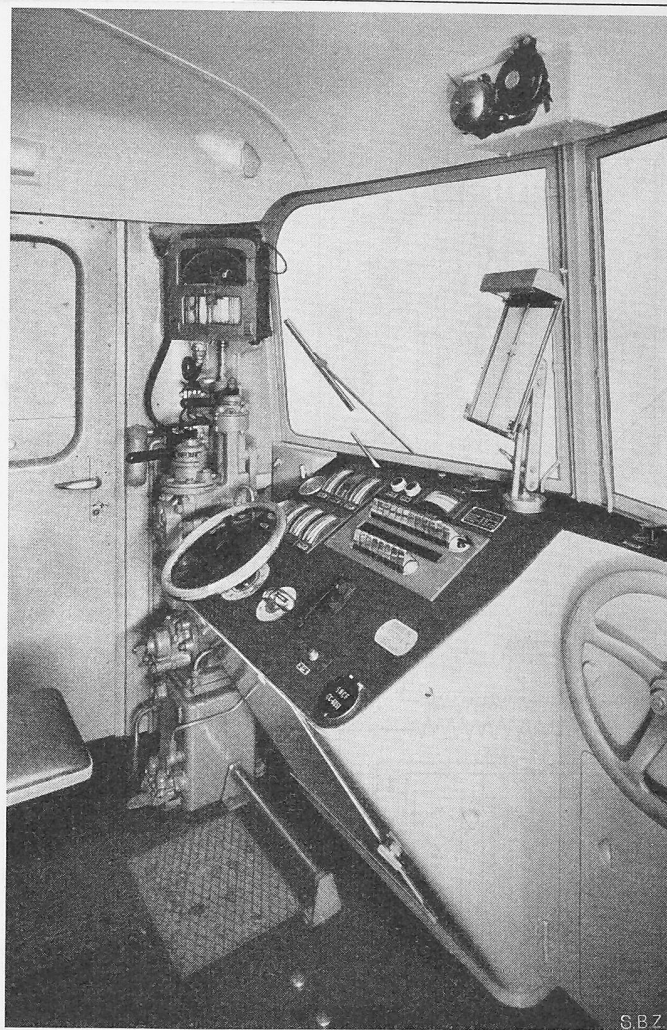
Bild 19. Führerstand der C 0 C 0 -Lokomotive
