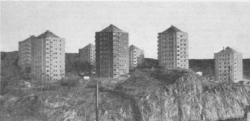
Bild 18. Hochhäuser auf Granitfels in Stockholm, sog. Punkthäuser. Die Wände bestehen aus 15 cm Massivbeton und 10 bzw. 12,5 cm (Nordseite) Siporexisolierung; farbiger Verputz. Architektonische Gestaltung umstritten.
