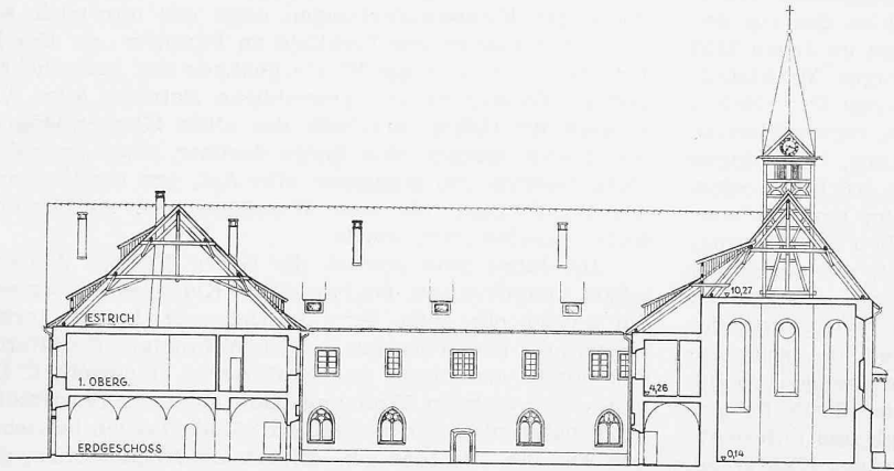
QUERSCHNITT DURCH NORDFLÜGEL
