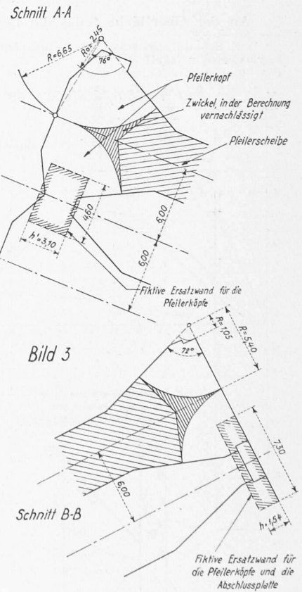
Hauptabmessungen und schematische Darstellung der untersuchten Konstruktion
