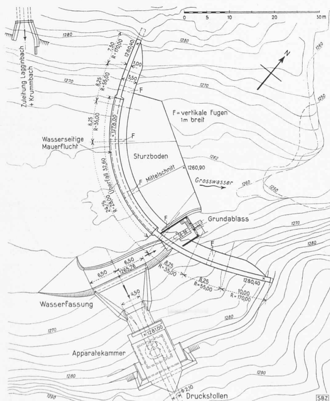
Bild 1. Situationsplan; 1: 800
