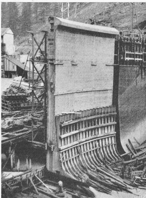
Bild 9 (links). Mauerelement in Mauermitte
