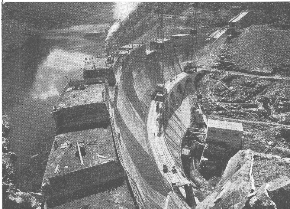
Staumauer Forte Buso, 140 000 m 3 Frioplast-Beton (die ersten 120 000 m 3 wurden mit einem gewöhnlichen Air-entrainer ausgeführt)
