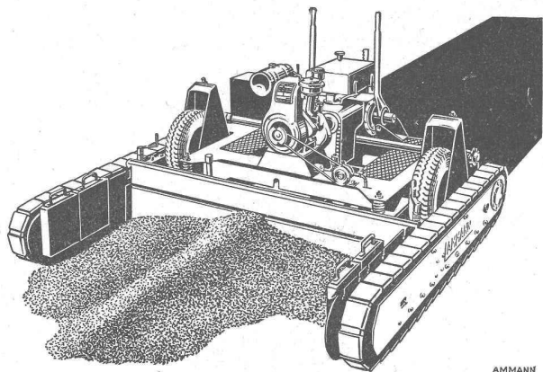
Einbaumaschine auf Raupen zum Einbauen von Warm- und Kaltbelägen Einäubreite einstellbar bis 2,05 m; Leistung bis 300 m 2 /h
