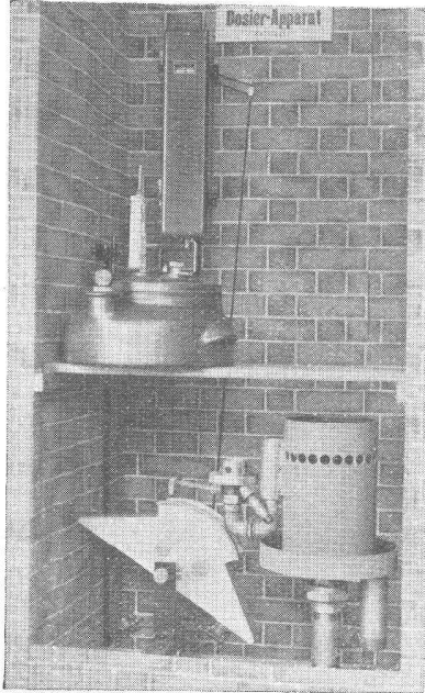
Ausführung mit Wippe für mechanische Steuerung
