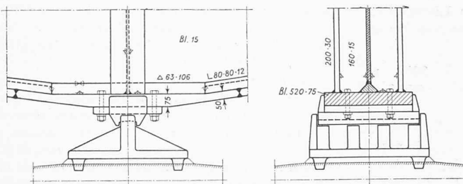
Bild 8. Querschnitt der Brücke 1:80
