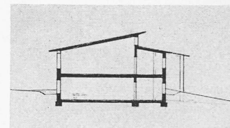
Querschnitt Masstab 1:600
