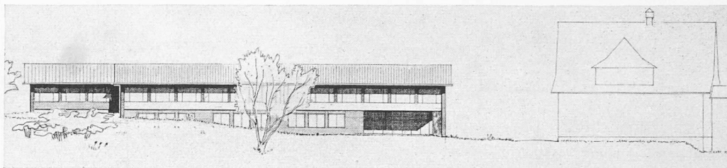
Südostansicht Masstab 1:600
