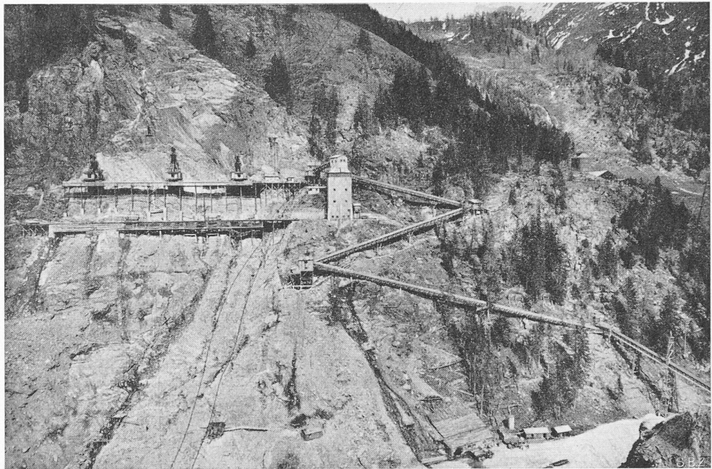
Bild 15. Betonaufgabe (17), Betonturm (16), Förderbänder (13)
