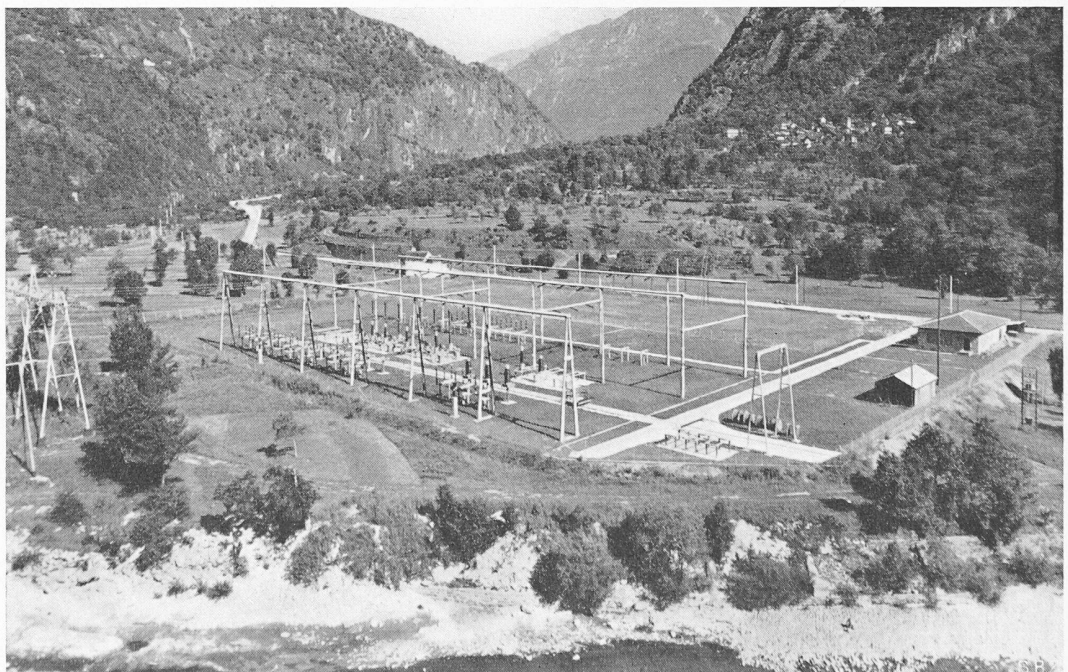
Bild 22. Schaltstation Avegno, im Vordergrund die Maggia
