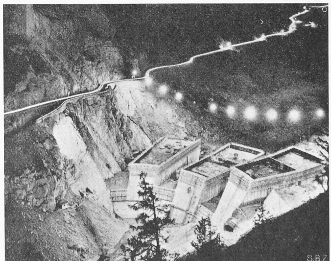
Bild 16. Aufbereitungsanlage (12), im Hintergrund der Stauraum von Sambuco
