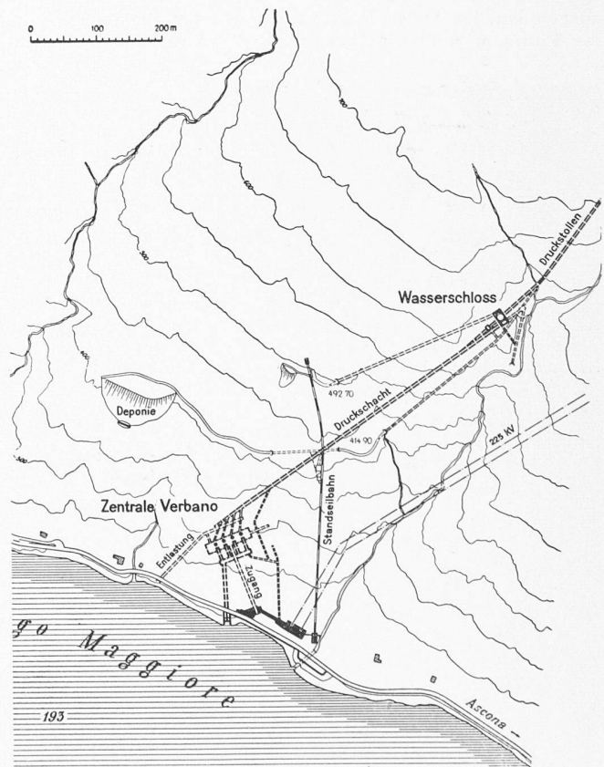
Bild 9. Wasserschloss, Druckschacht und Zentrale Verbano, Plan 1: 10 000
