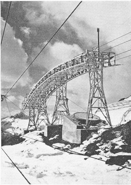
Bild 21. Luftseilbahn für den Zementtransport Rodi-Sambuco, Uebergangsstation Campolungo
