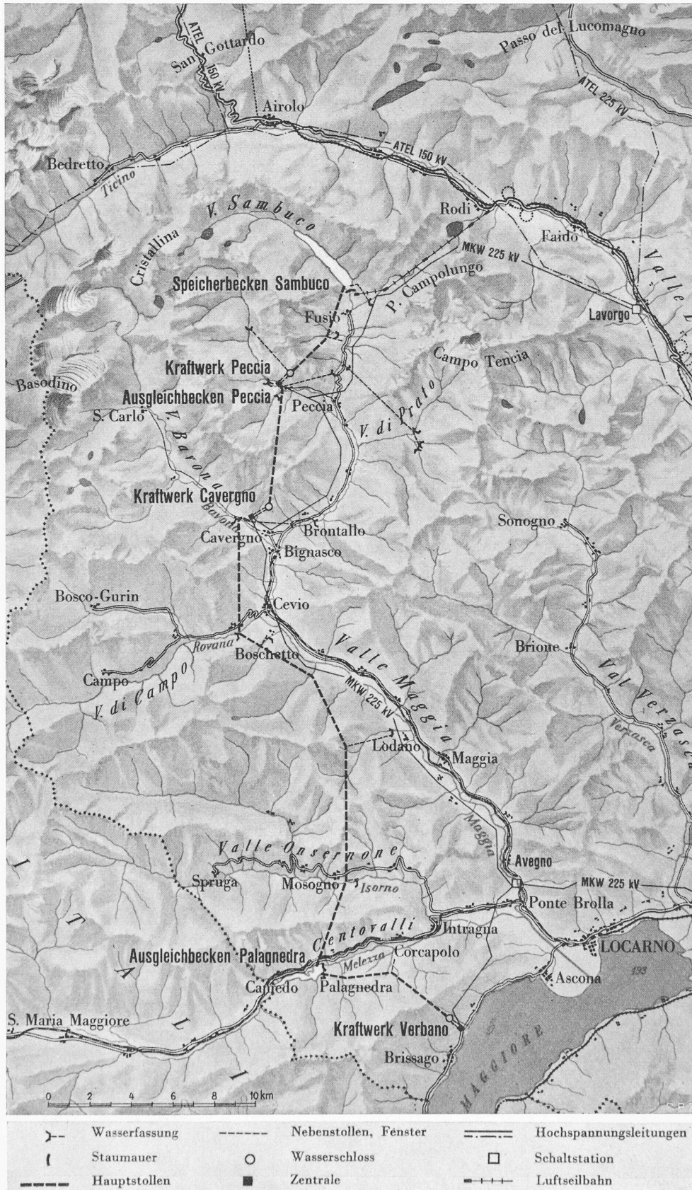
Bild 2. Maggia-Kraftwerke, Uebersichtskarte 1: 250 000
