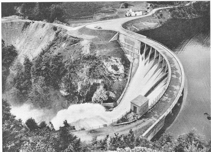
Bild 8. Staumauer Palagnedra, Ueberfall am 30. Juni 1953
