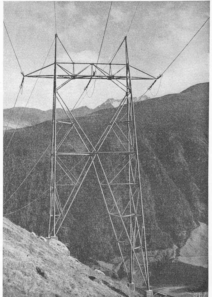
Bild 3. 380 kV-Abspannmast der Lukmanierleitung
