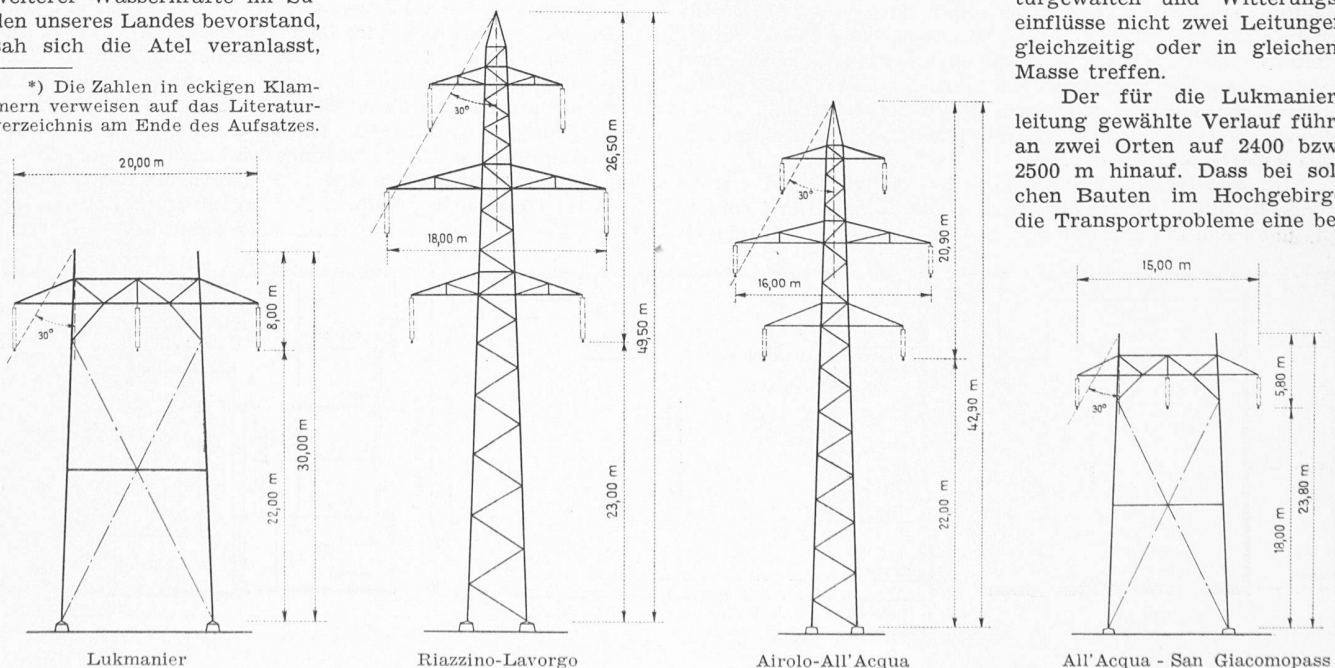
Bild 1. Ausbetonierte Rohrgittermaste von Hochspannungsleitungen der Aare-Tessin AG. (Tragmaste). Masstab 1:600
