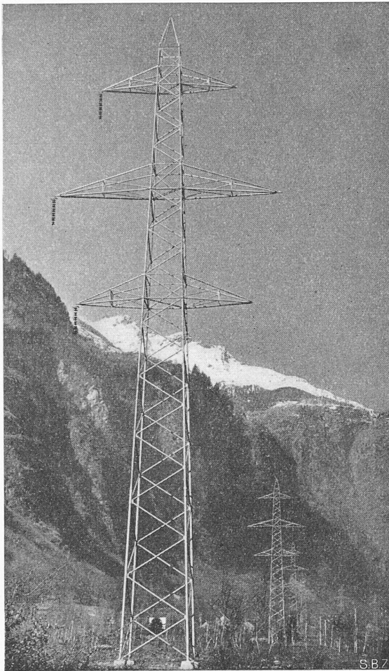
Bild 4. 330 kV-Tragmast der 225 kV-Leitung Riazzino-Lavorgo
