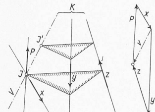
Bild 1. Die bekannte Kraft P schneidet sich mit der Wirkungslinie einer unbekannt Kraft x zugänglich im Punkt J .
