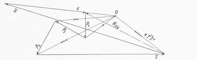
Bild 4. Ermittlung der Stabkräfte eines ebenen Fachwerkes nach der Schnittmethode für den Fall, dass kein Schnittpunkt zweier Stabrichtungen auf dem Zeichenblatt liegt (Seileckverfahren).
