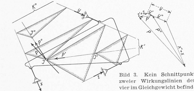
Bild 3. Kein Schnittpunkt zweier Wirkungslinien der vier im Gleichgewicht befindlichen Kräfte liegt auf dem Zeichenblatt.
