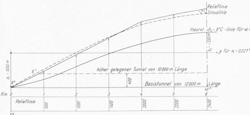
Bild 4. Schematisches Beispiel für h/l = 1/10
